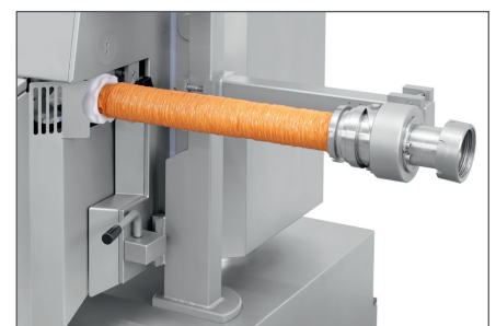
Tête pivotante pour une utilisation universelle.
