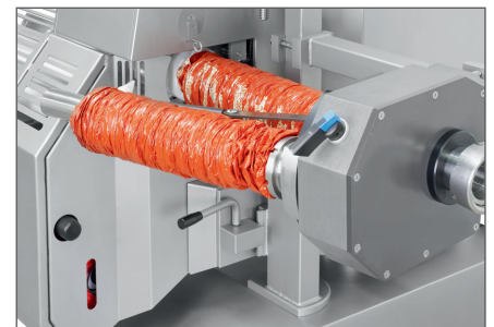
Deux systèmes de revolver : tourelle revolver en V ou tourelle parallèle pour un changement de boyau rapide.
