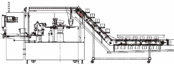
• 搭配碗型輸送帶，投入固型物再搭配液體充填機
