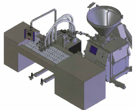
(C) 搭自動成型製袋包裝機
