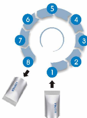
(A) 搭配給袋式包裝機 (各式袋子) 自動取袋→開袋→充填→封口
